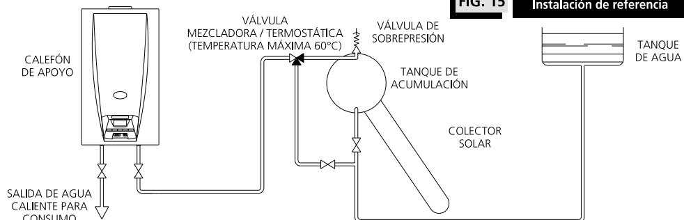
FIG. 15 Instalación de referencia
